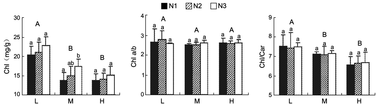
图 2 不同光强和施氮处理下的光合色素
